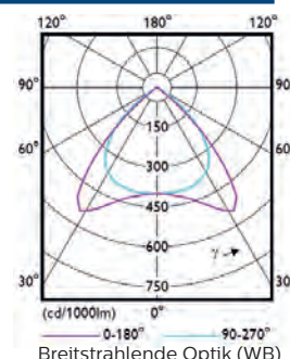
Breitstrahlende Optik (WB)
