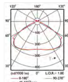
VWB (sehr breitstrahlend)
