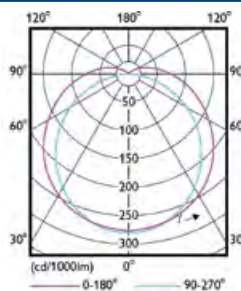
WT120C G2 PSU
