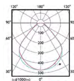
SP402P, direkt, quadratisch
