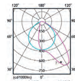
SM544C, asymmetrisch
