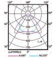
Breitstrahlend (WB)
