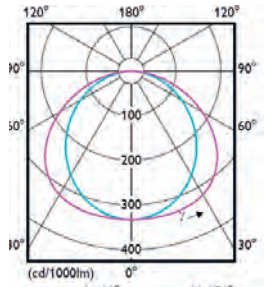
RC132V/RC133V NOC
