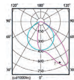
SM534C, asymmetrisch
